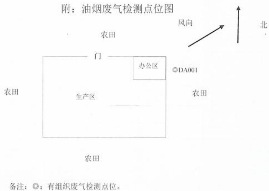
图7-2 东厂区食堂油烟监测点位示意图
